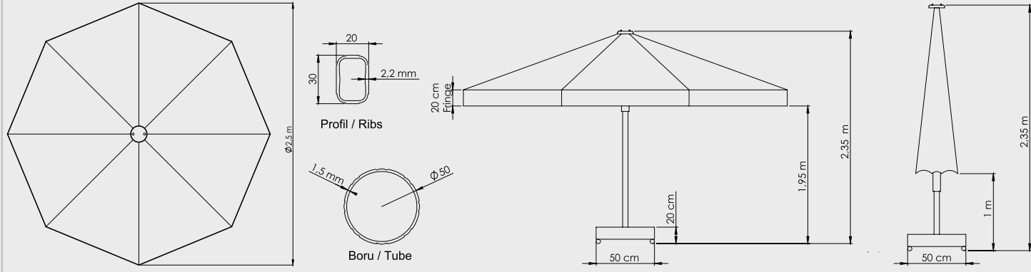
Avokado Klips Yuvarlak 250/8 Avocado Clips Circular 250/8
