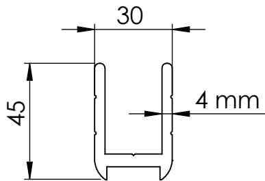
Mafsal / Hinge
