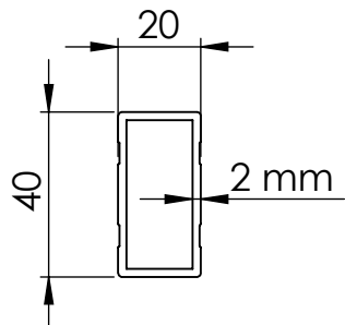
Profil / Rib
